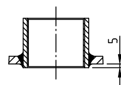
Muffeneinschweißung Entlüftungs-u. Abbläsmuffe innen bündig
